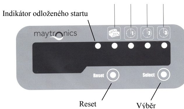
Kontrolka plného filtračního sáčku – orientační LED1 LED2 LED3
